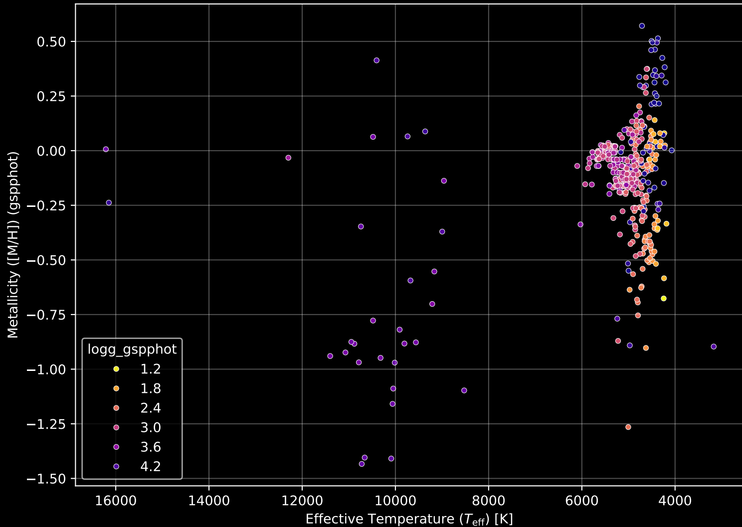
APOGEE DR17 Field: [195+08] Stellar Population Parameters (n= 445)
